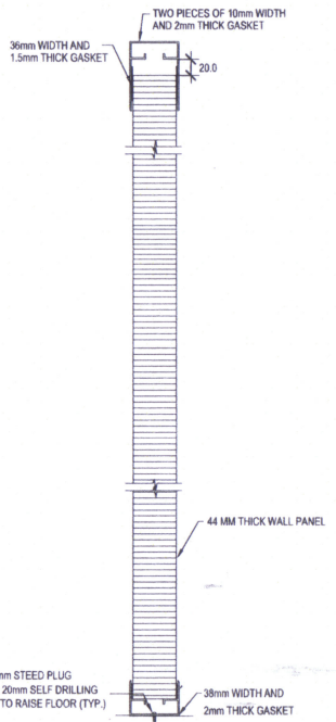
7 VERTICAL WALL SECTION SCALE: N.T.S.
