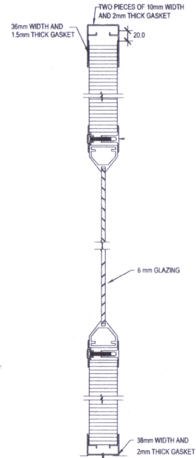
8 VERTICAL WALL SECTION W/ WINDOW SCALE: N.T.S.
