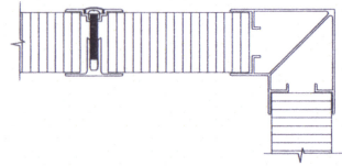
4 HORIZ. WALL SECTION W/ CORNER POST SCALE: N.T.S.
