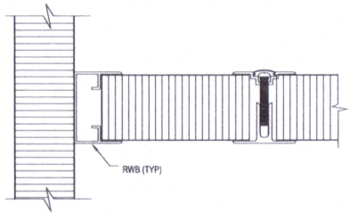
3 HORIZONTAL WALL SECTION MEETING PANEL SCALE: N.T.S.
